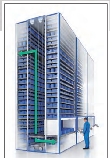
Hänel Lean-Lift® mit Vertikal-Technik – das Original mit der Hänel Rasterwand®
